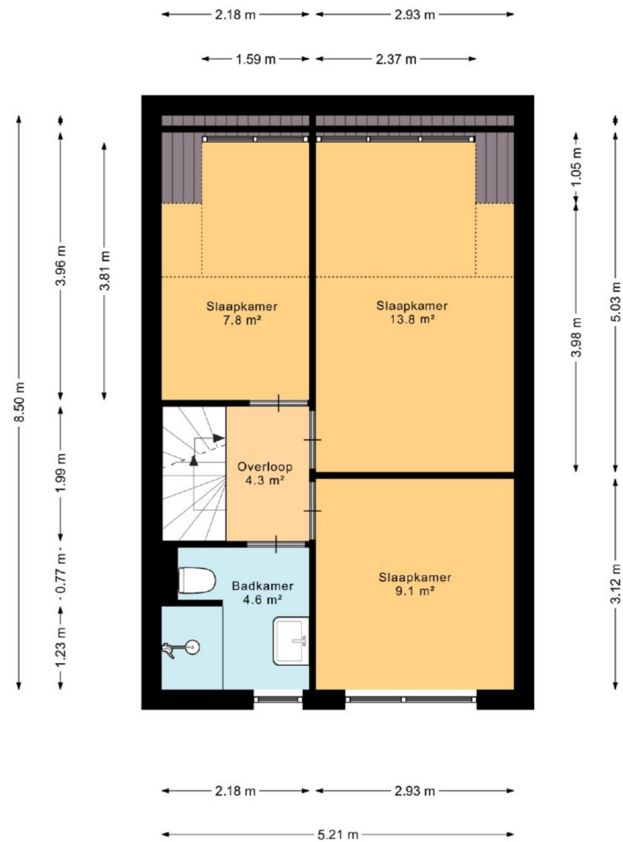
1e Verdieping
